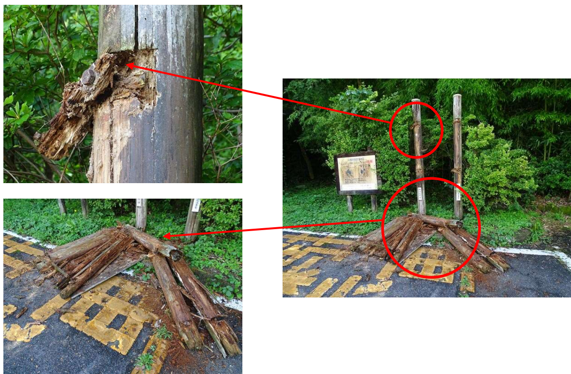
写真 3：市営板室駐車場 看板 D「D 判定」（全面腐朽）
