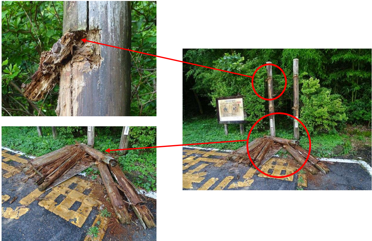
写真 3：市営板室駐車場 看板 D「D 判定」（全面腐朽）
