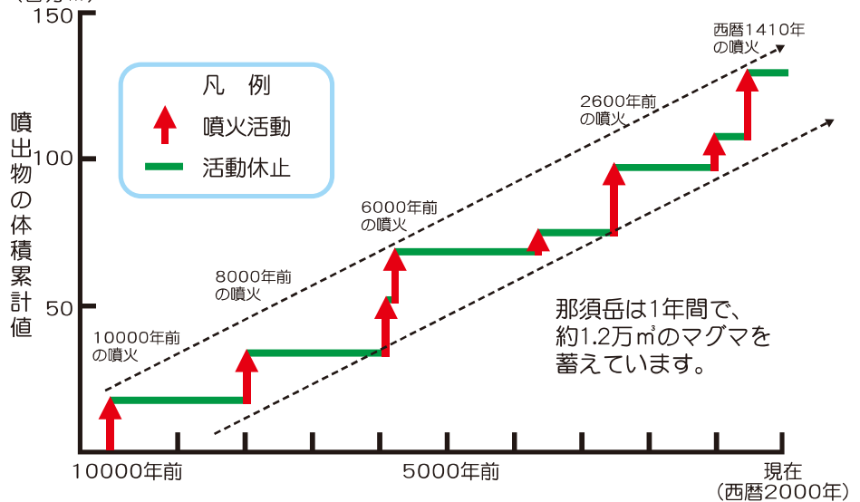
(百万m 3 ) 那須岳（茶臼岳）の過去1万年の噴火活動（階段ダイヤグラム）
