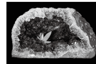
紫水晶と方解石(栃木県立博物館蔵)
