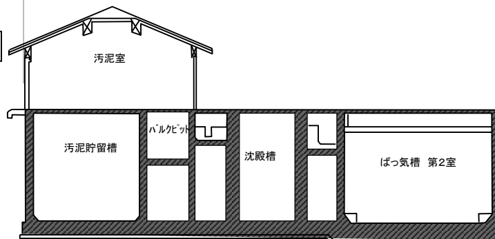
断面図
