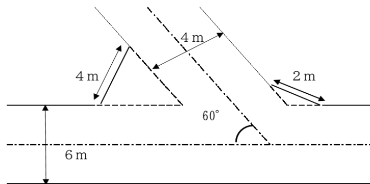
【隅切り例】
