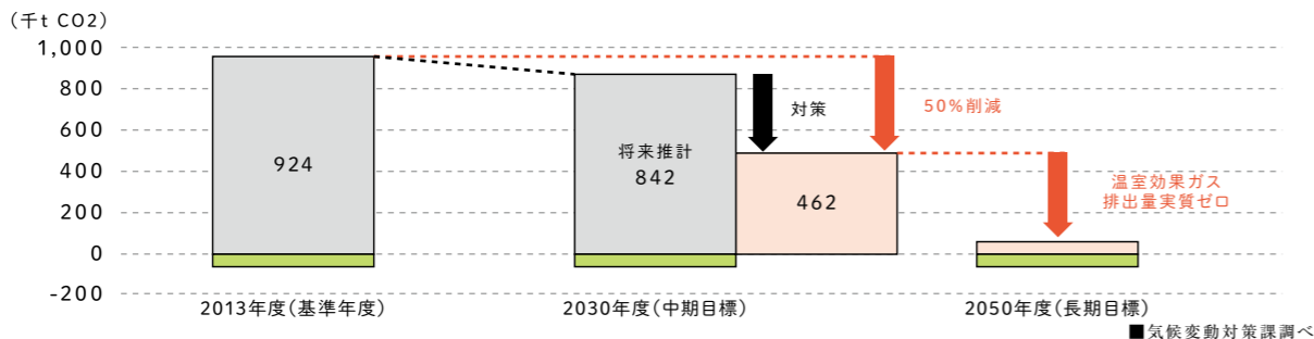
⇒ 温室効果ガス排出量の削減イメージ □温室効果ガス排出量 ■森林吸収量
