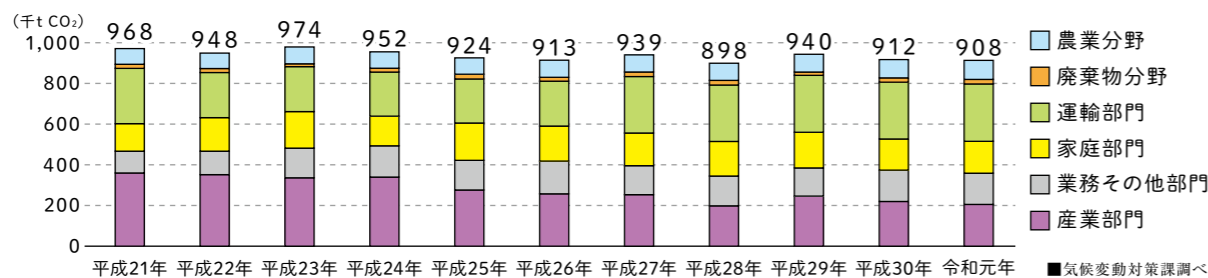
⇒ 本市の温室効果ガス排出量 ※平成30年、令和元年のデータは速報値
