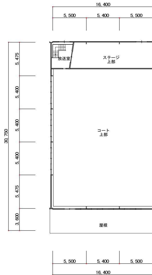
上部平面図 S = 1/300
