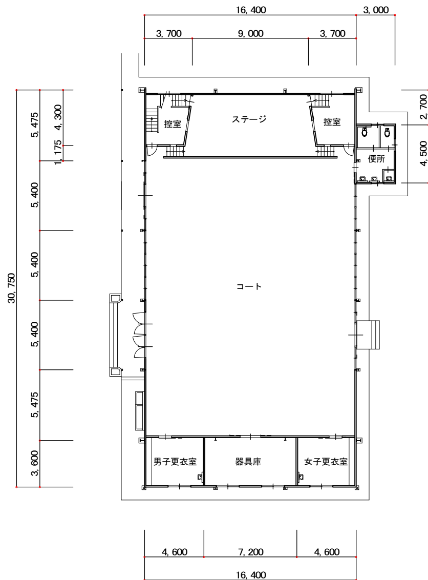
1階平面図 S = 1/300
