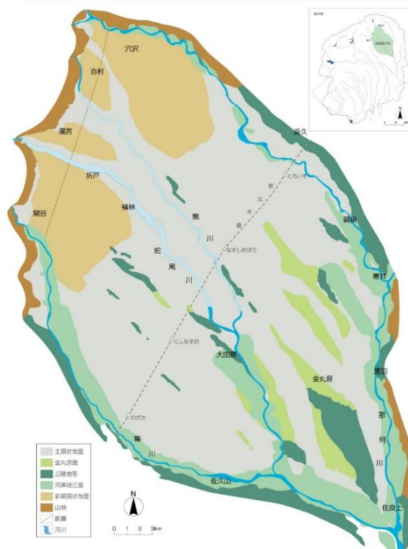
那須野が原扇状地の地形図
