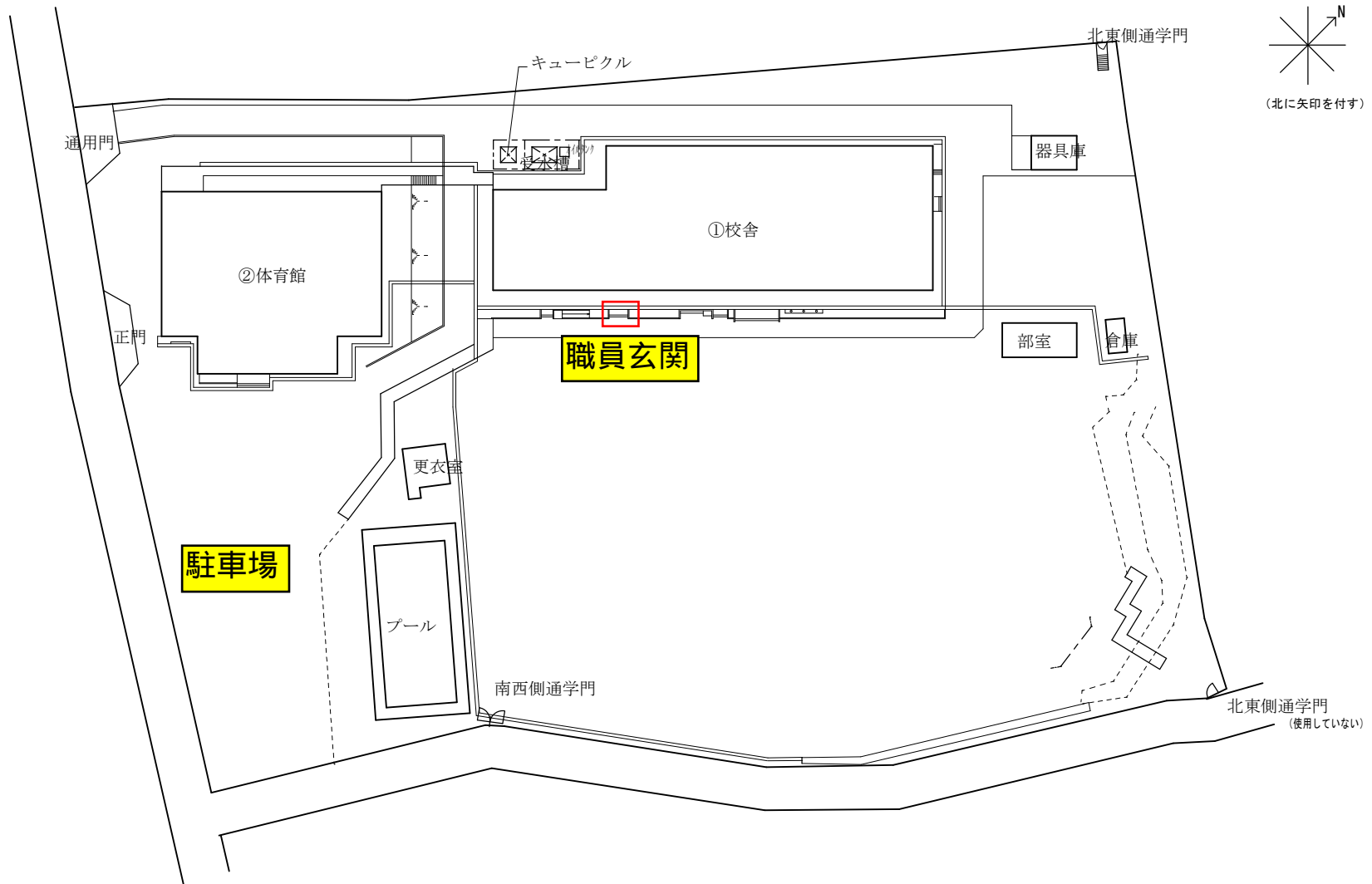
配置図 1/1000
